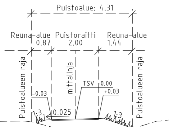
Tyyppipoikkileikkaus plv 5-23 (pl 16) 1:100
